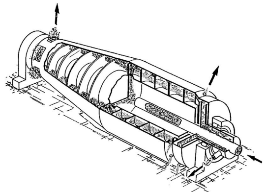
图 1 三相离心机结构示意图
